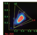
709/2020色域分布图
