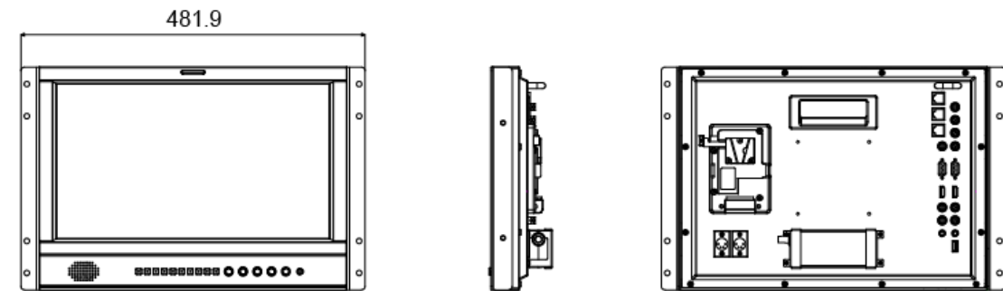
整机+边架
