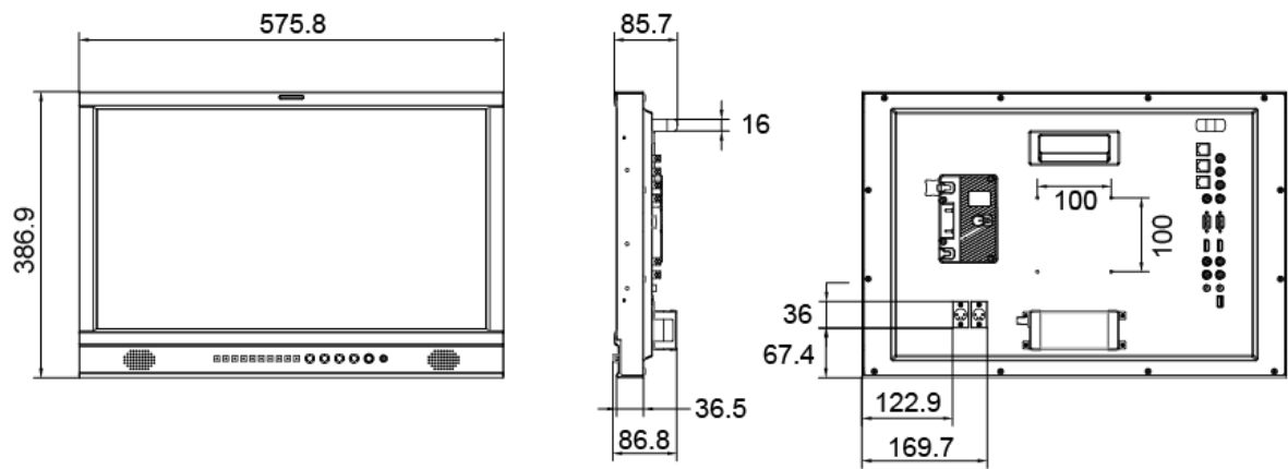
监视器+桌面支撑底座（单位：mm）
