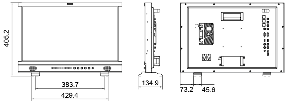
监视器+桌面支撑底座（单位：mm）
